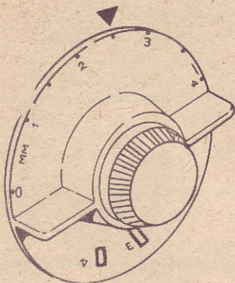
Tarcza długości ściegu
