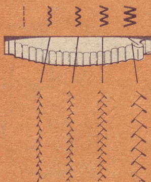
Nastawienie szerokości ściegu
